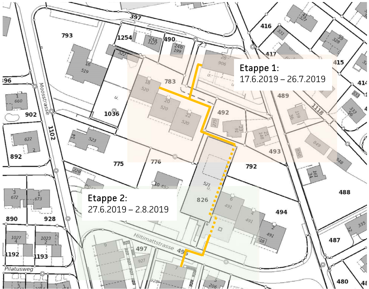
Abb 1: Übersichtsplan Etappierung Tiefbauarbeiten
